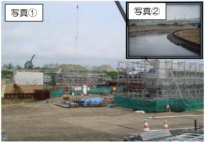
写真① 貞山運河にて捨石投入、川表基礎構築を継続しています。新仙流橋建設においては橋台・橋脚が完成し上部施工への準備を実施します。七ヶ浜町水路取替工事も継続しています。
