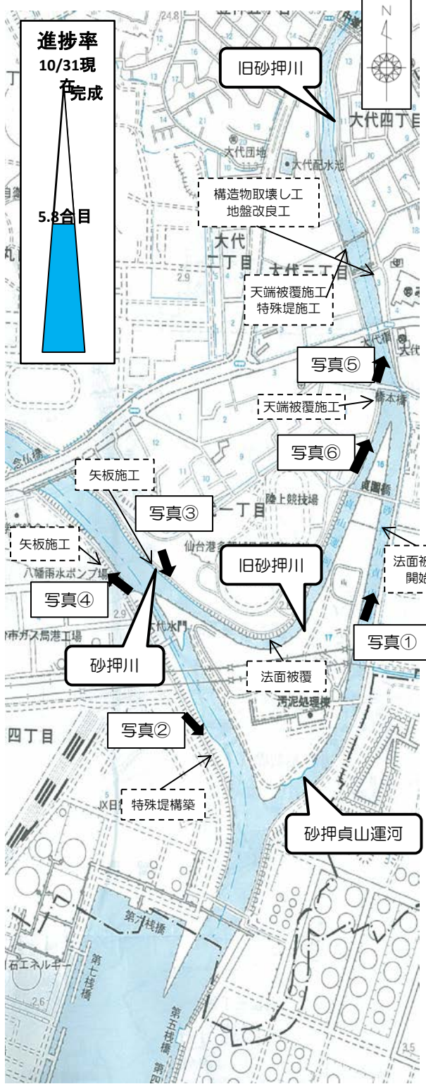
貞山運河では盛土と法面被覆工を開始し、旧砂押川では法面被覆工を継続しています。砂押川では捨石工と特殊堤（壁堤防）構築を継続しています。
