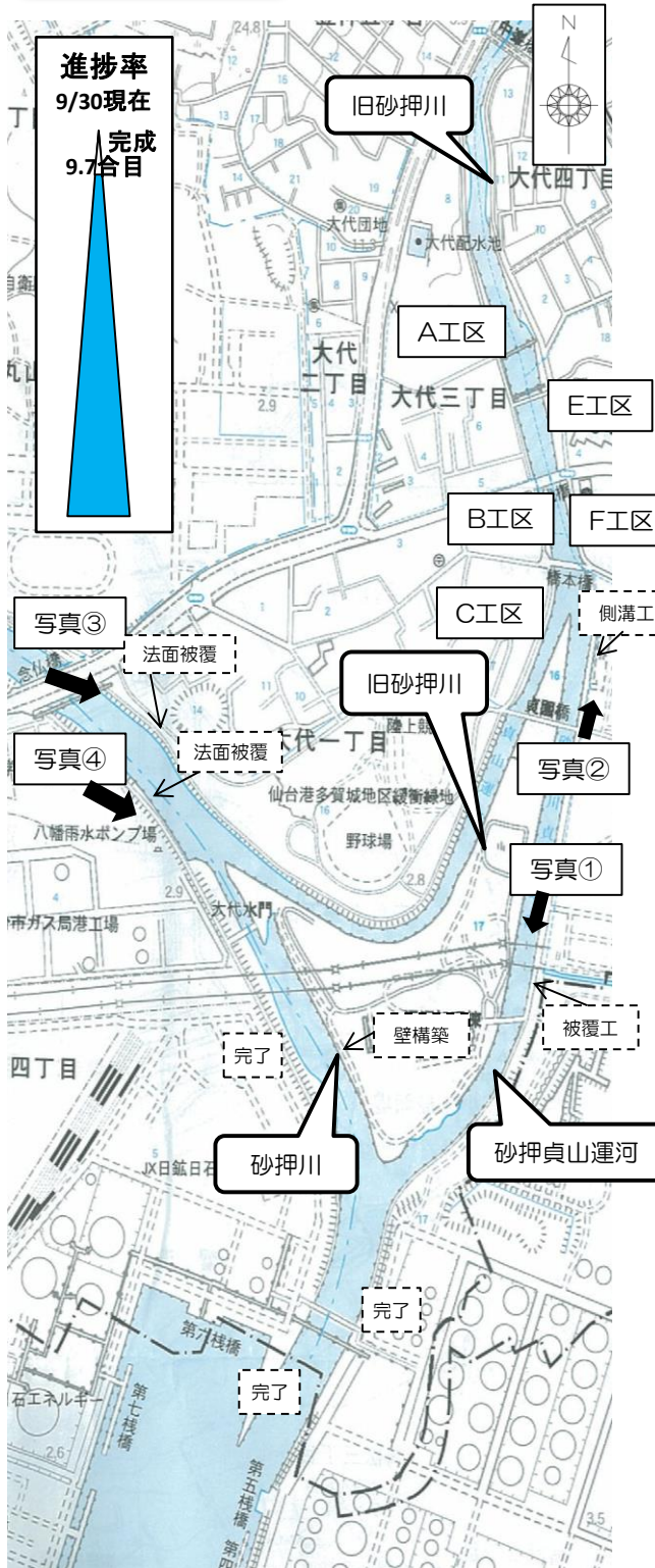
砂押川、貞山運河、旧砂押川の各所にて、新護岸としての被覆工と壁構築を継続で進めています。多賀城市道においては、片側交互通行にて道路側溝工事を継続で行っております。
