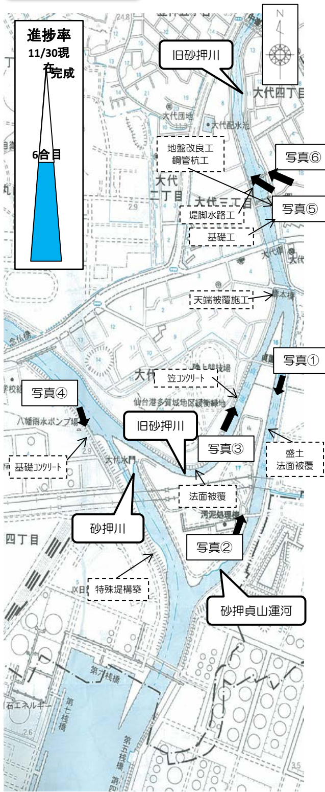
貞山運河では盛土と法面被覆工を継続し、旧橋撤去も進めています。旧砂押川では法面被覆工を継続、砂押川では捨石工と特殊堤(壁堤防)構築を継続しています。
