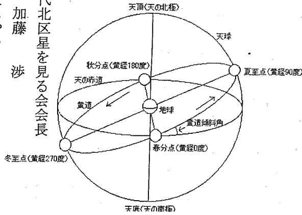
上図は、黄道と黄径を表示し地球の傾き角度による太陽運動を示した物地球を静止にした状態
