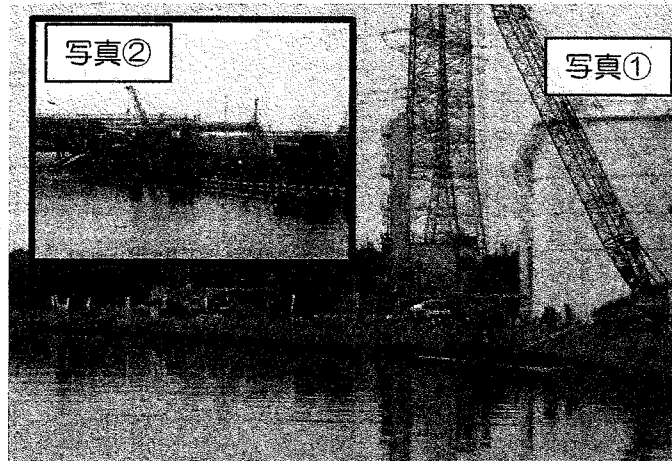
写真① 中洲・JXエリアにて崩れた構造物撤去と、鋼矢板打設を行っています。10月から、市道を仮設道路への切り替え、海上部(象の鼻)では海上クレーンによる構造物撤去作業を開始しました。
